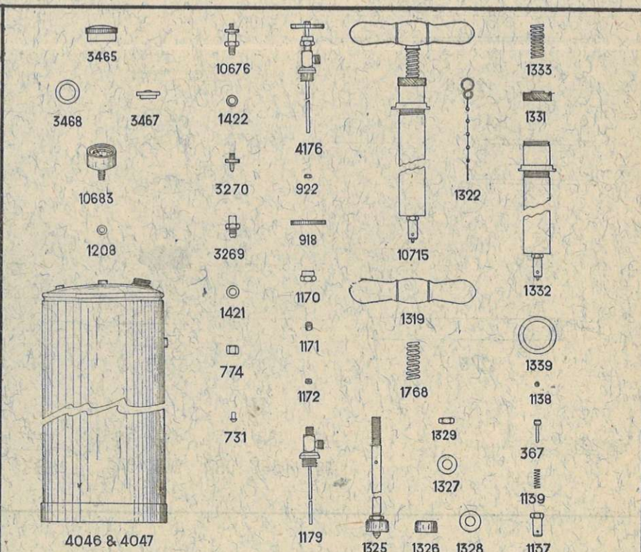
Réservoirs essence à pression - Pressure containers for petrol Depositos a presion para gasolina
