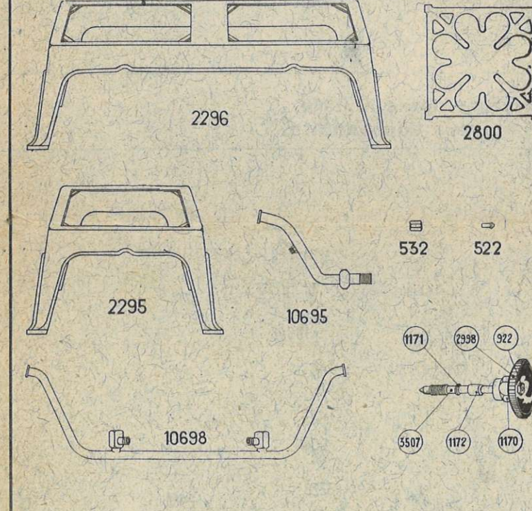
Réchauds pétrole pour réservoirs indépendants Paraffin stoves fed by se separate container Hornillos de cocina a petroleo con deposito separado
