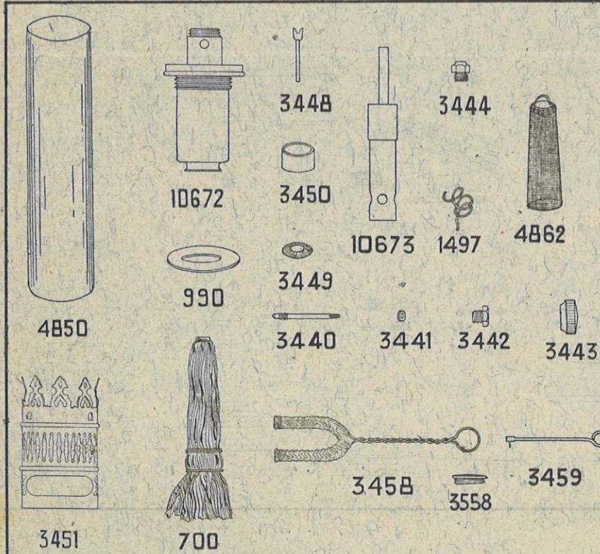
Bec droit N° 4800 à essence sans pression Straight burner N° 4800 working with petrol without pressure Mechero recto N° 4800 a gasolina sin presion
