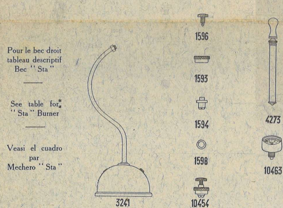
Lampe de table N° 1965 Swan neck lamp - Lampara de mesa
