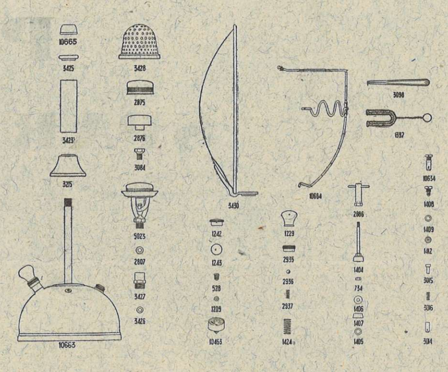
Radiateur pétrole N° 5046 Paraffin radiator - Radiador a petroleo
