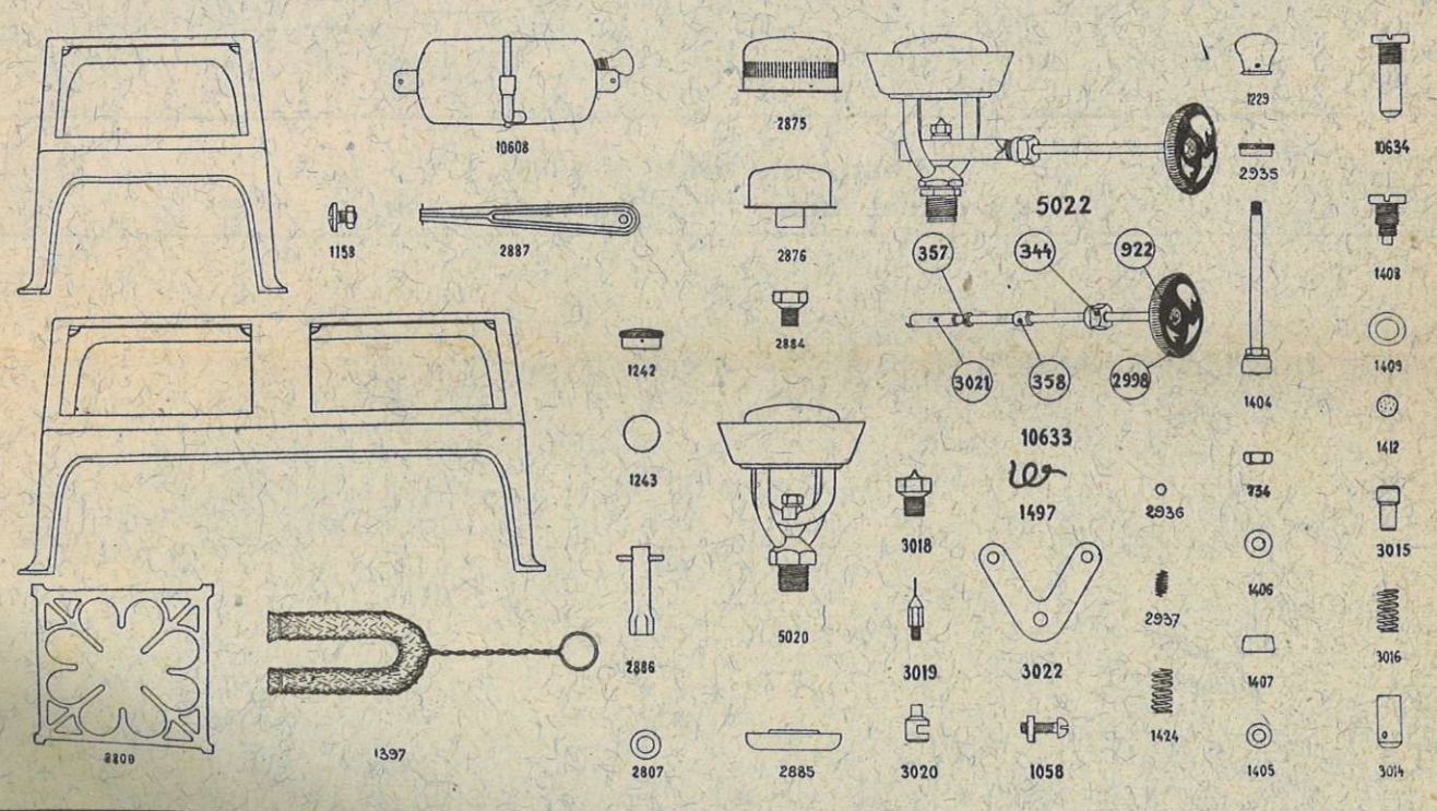
Réchauds pétrole N° 5003, 5004, 5005, 5006 Paraffin cooking rings - Hornillos a petroleo
