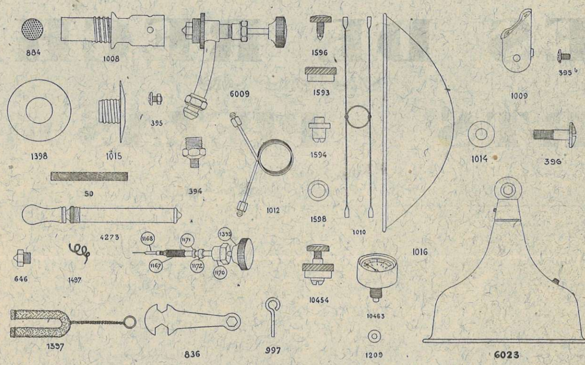
Radiateur essence N° 4062 Petrol radiator - Radiador a gasolina
