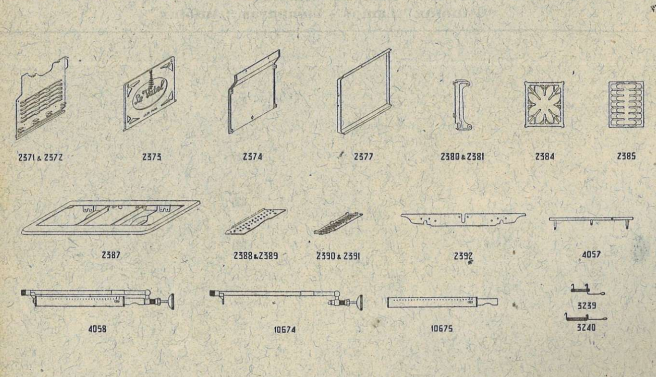
Grilloir-Rôtissoire Four N° 5066 à essence pour réservoir indépendant Petrol grilling and roasting Range 5066 fed by separate container Horno tostador asador a gasolina con deposito separado
