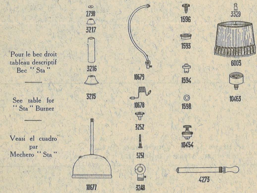
Lanterne Tempête N° 5080 Hurricane lantern - Linterna huracan
