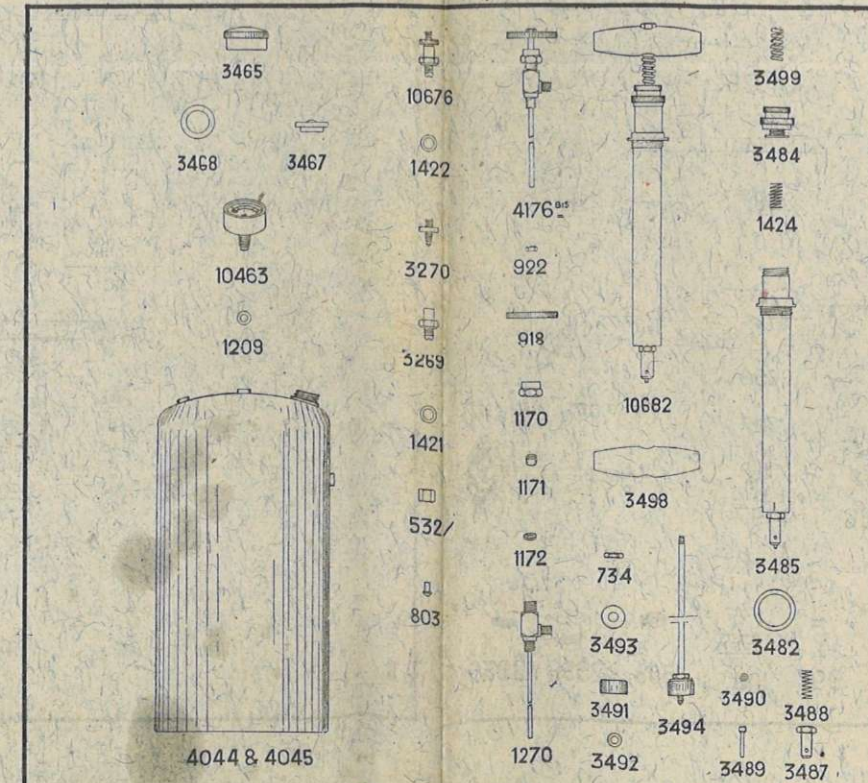
Réservoirs essence à pression - Pressure containers for petrol Depositos a presion para gasolina
