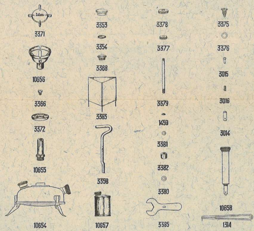
Réchaud pétrole démontable N° 5017 Paraffin camp stove - Infiernillo a petroleo
