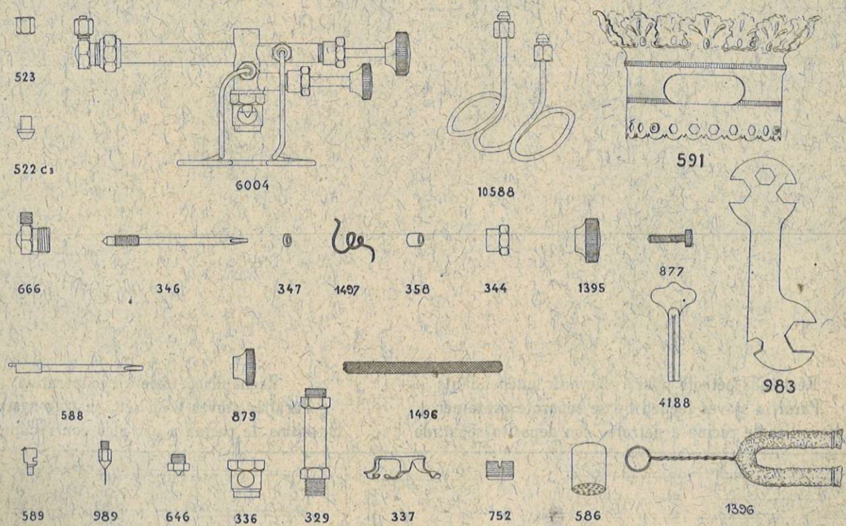
Lampe à réflecteur dôme N° 1960 Dome Lamp - Lampara con pantalla
