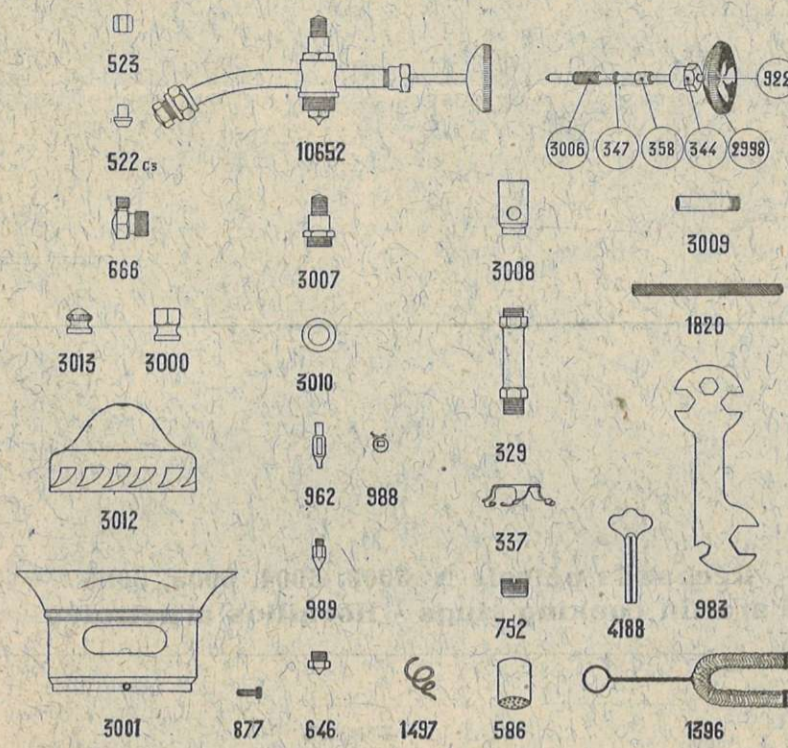
Lampe de table N° 1965 Swan neck lamp - Lampara de mesa
