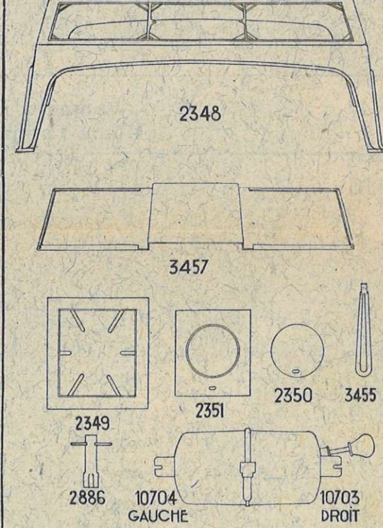
Réchauds pétrole à récupération Paraffin stoves with self heating system Hornillos de cocina a petroleo con recuperacion
