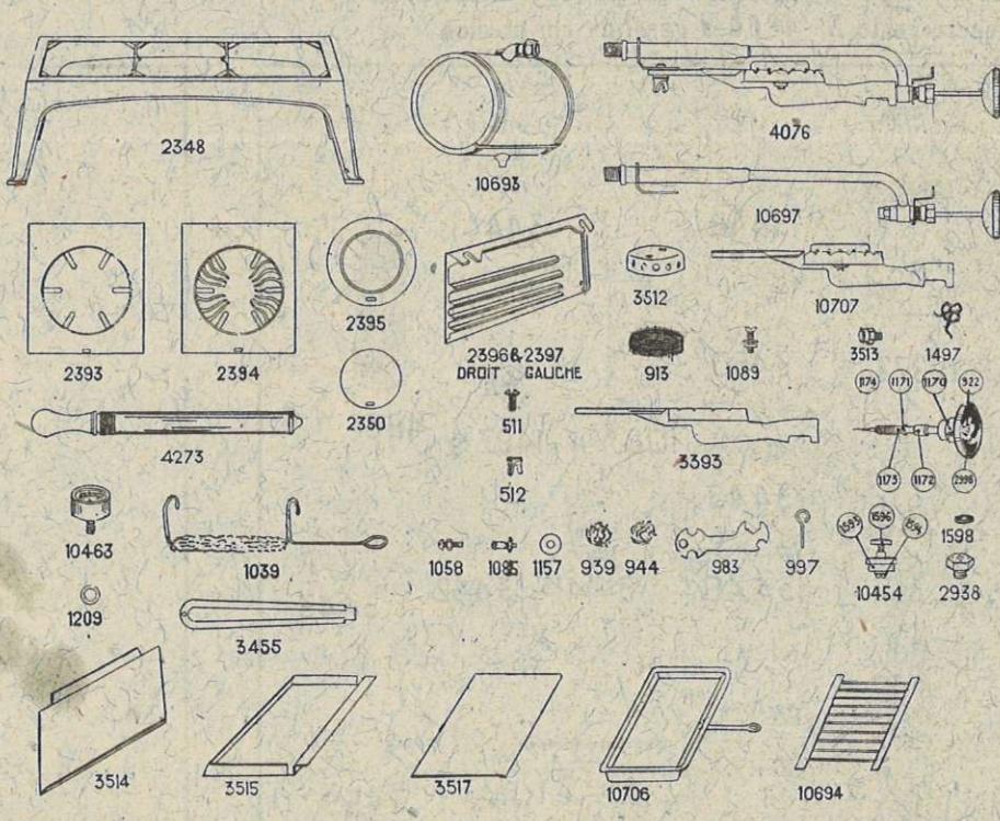
Réchaud grilloir à essence Petrol grilling stove - Horno tostador à gasolina
